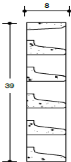
CORTE AA
