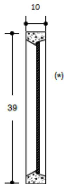
CORTE AA
